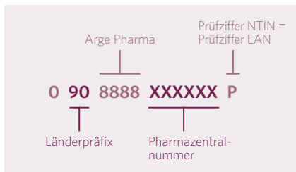
Abbildung 6: Aufbau NTIN mit führender „0“ für GS1 Data Matrix Code, basierend auf dem EAN-13 Code
